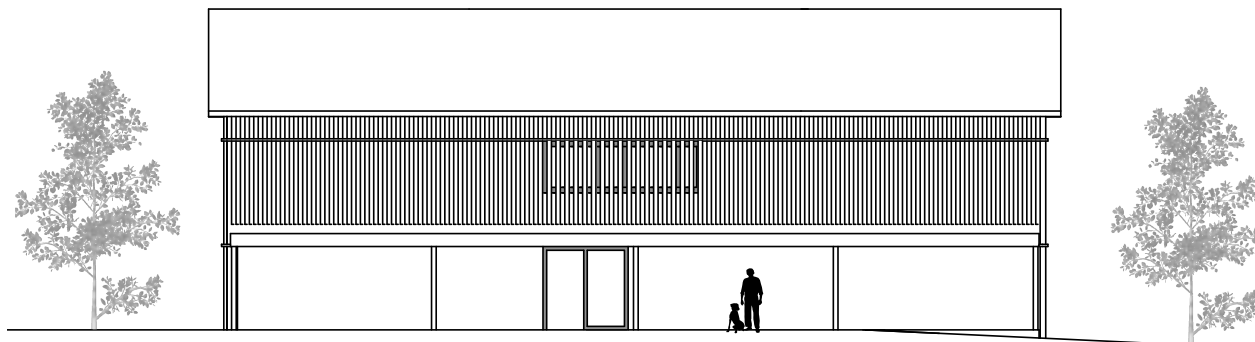
ANSICHT NORD
