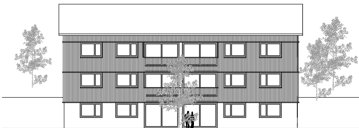
ANSICHT SÜD
